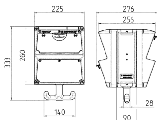
Чертеж 1 MB 630
