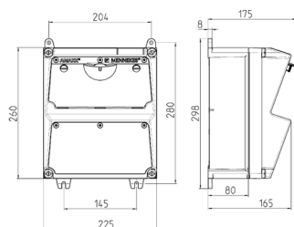
Чертеж 1 МВ 521
