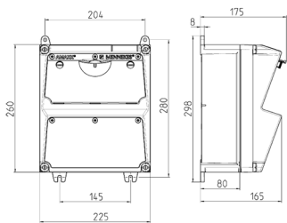
Чертеж 1 MB 521
