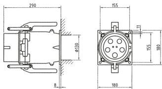
Чертеж 2 МВ 199/1 Размеры, мм.
