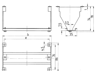
Чертеж 6 МВ 18
