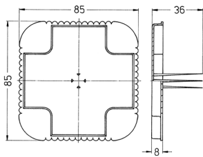
Чертеж 1 МВ 353 Размеры, мм.
