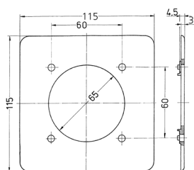
Чертеж 1 МВ 233 Размеры, мм.
