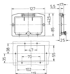
Чертеж 6 МВ 4 Размеры, мм.
